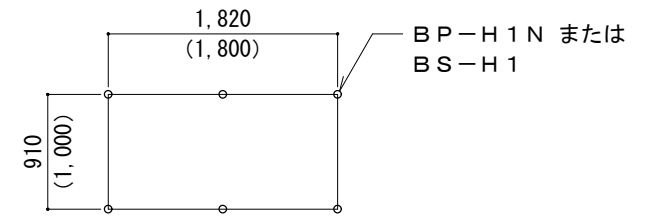
断熱材 仮固定ピッチ
