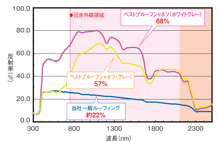
■図5 分光反射率グラフ(300nm~2500nm)
