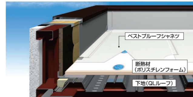
■図2 工場や倉庫などの金属下地屋根の例
