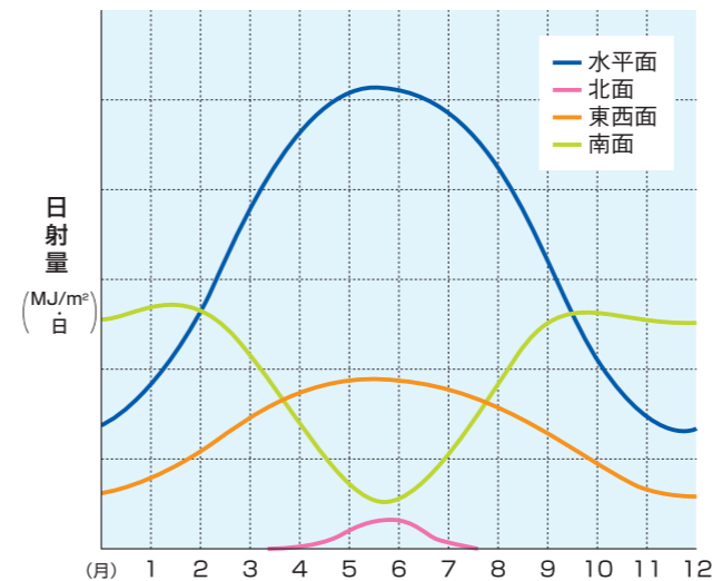
■年間の日射量
