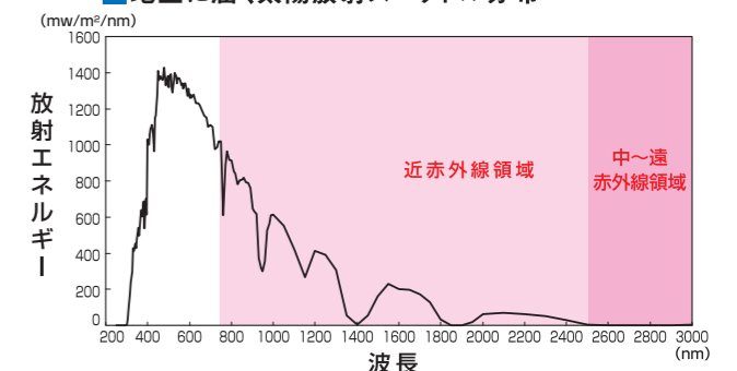
■地上に届く太陽放射スペクトル分布
